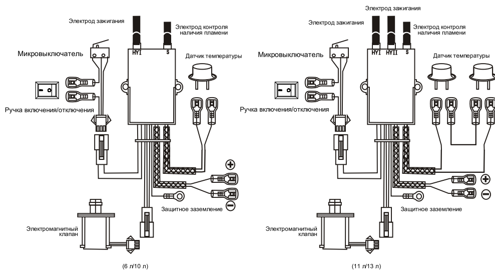
Принципиальная электрическая схема
