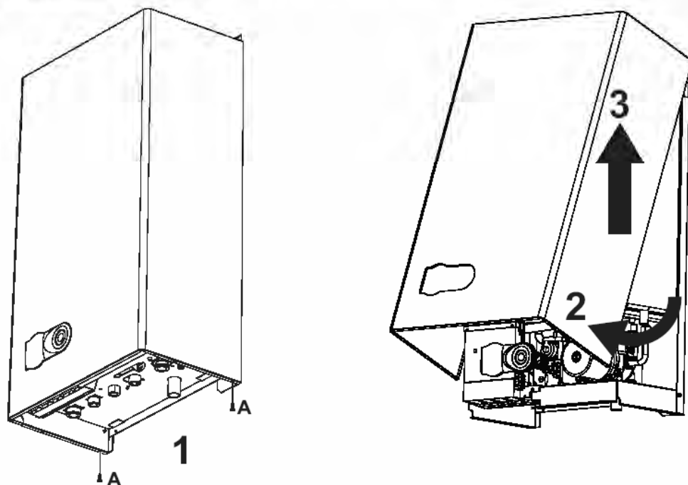
рис. 9 - Снятие кожуха
