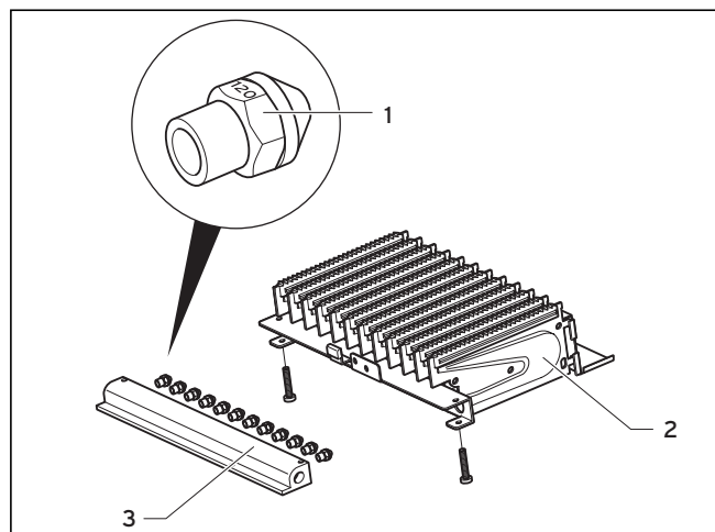
Рис. 6.4 Маркировка сопла
