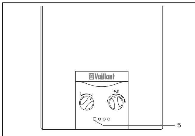
Рис. 7.10 Разблокировка
