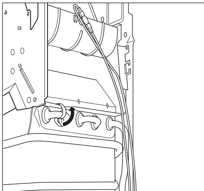
Рис. 7.8 Демонтаж теплообменника
