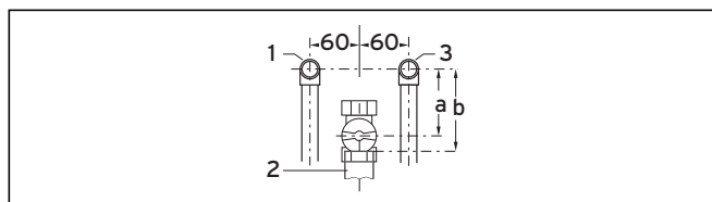
Рис. 4.3 Предварительный монтаж
