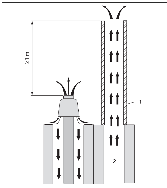
1 Насадка димаря
