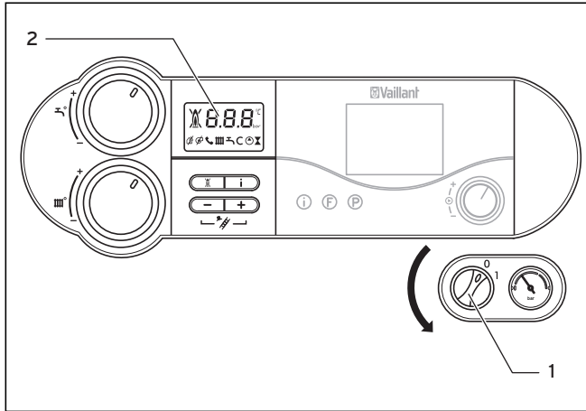
Рис. 4.14 Вимкнення приладу
