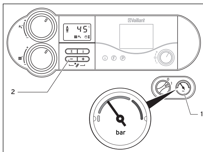
Рис. 4.13 Проверка давления напoлнения отопительной установки
