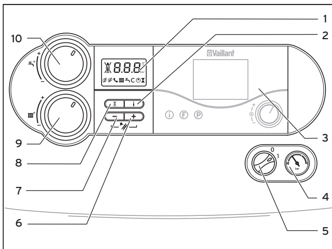
Рис. 4.2 Органи управління
