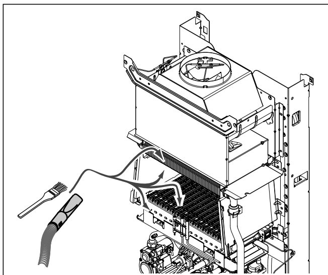
Мал. 8.1 Очищення палика і первинного теплообмінника без демонтажу деталей (незначне забруднення)
