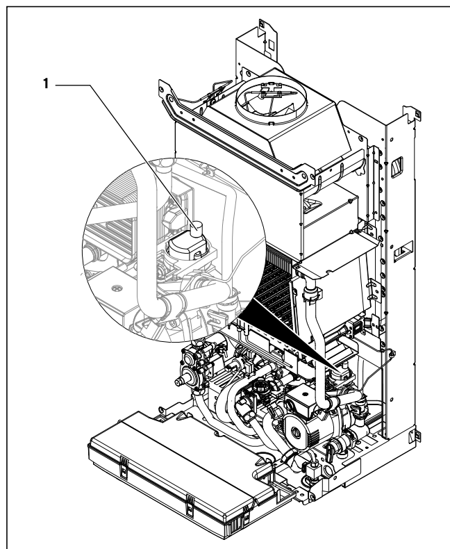
Рис. 6.1 Быстродействующий воздухоотводчик
