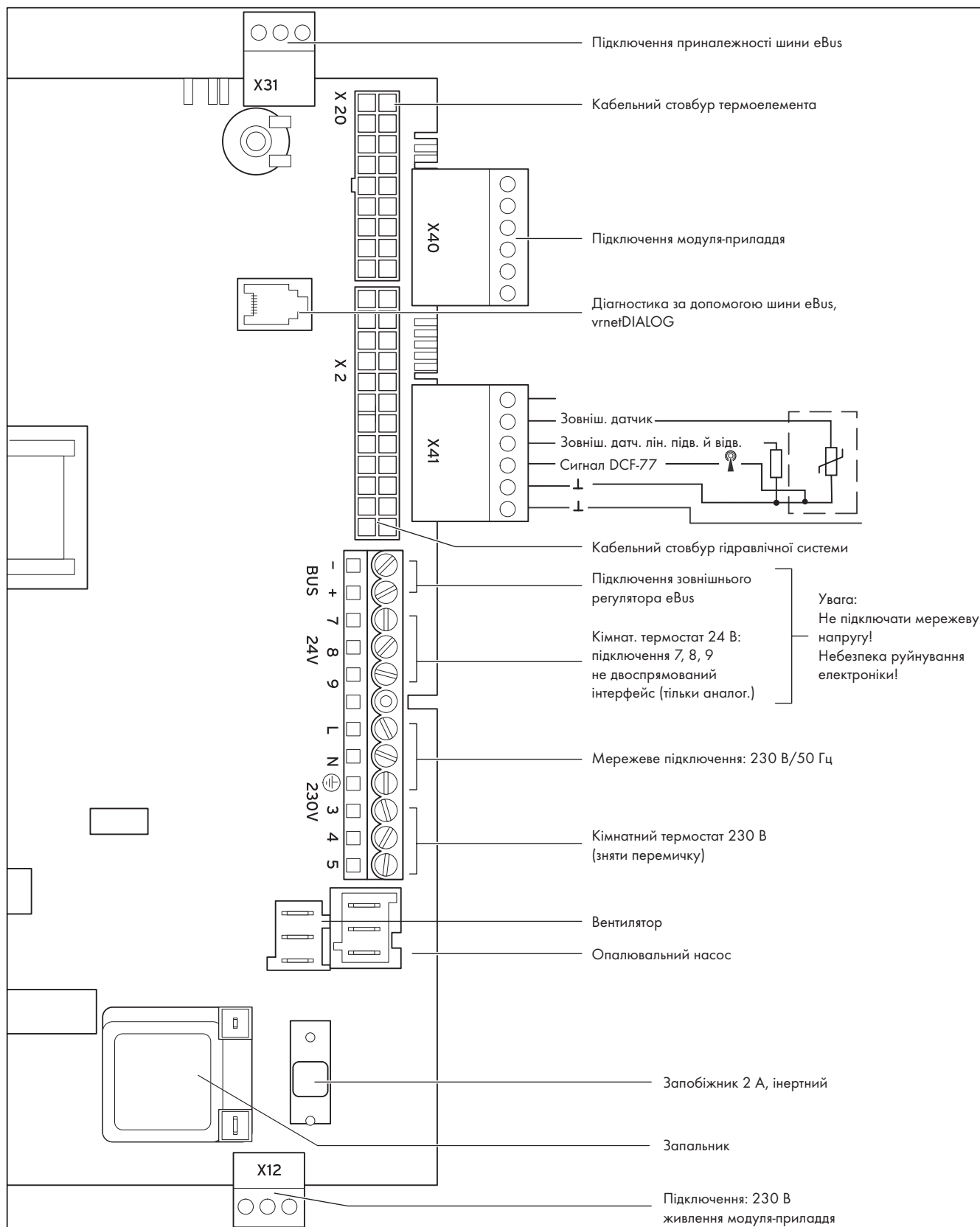
Мал. 5.8 Схема з'єднань turboTEC pro
