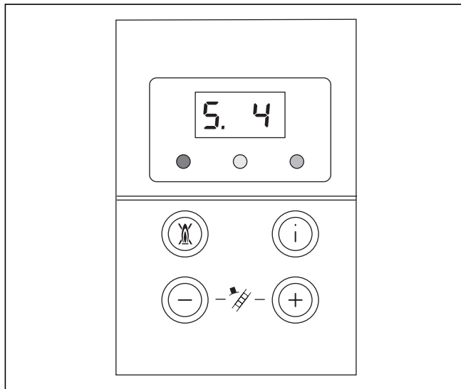
Мал. 6.6 Індикація на дисплеї в режимі опалення
