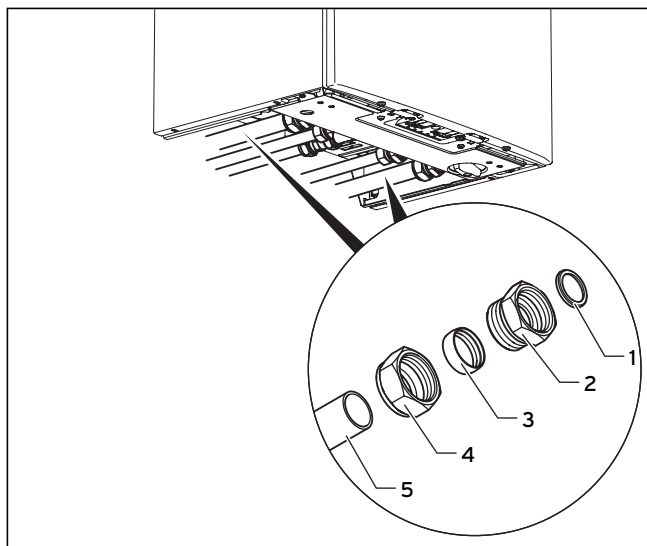
Мал. 5.3 Монтаж ліній подачі і зворотної лінії.
