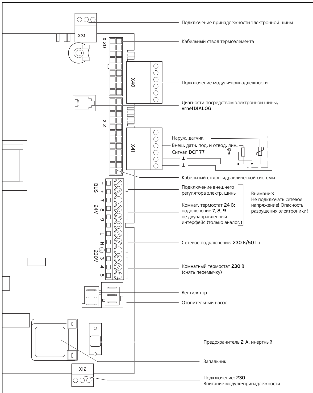
Рис. 5.8 Схема соединений turboTEC pro
