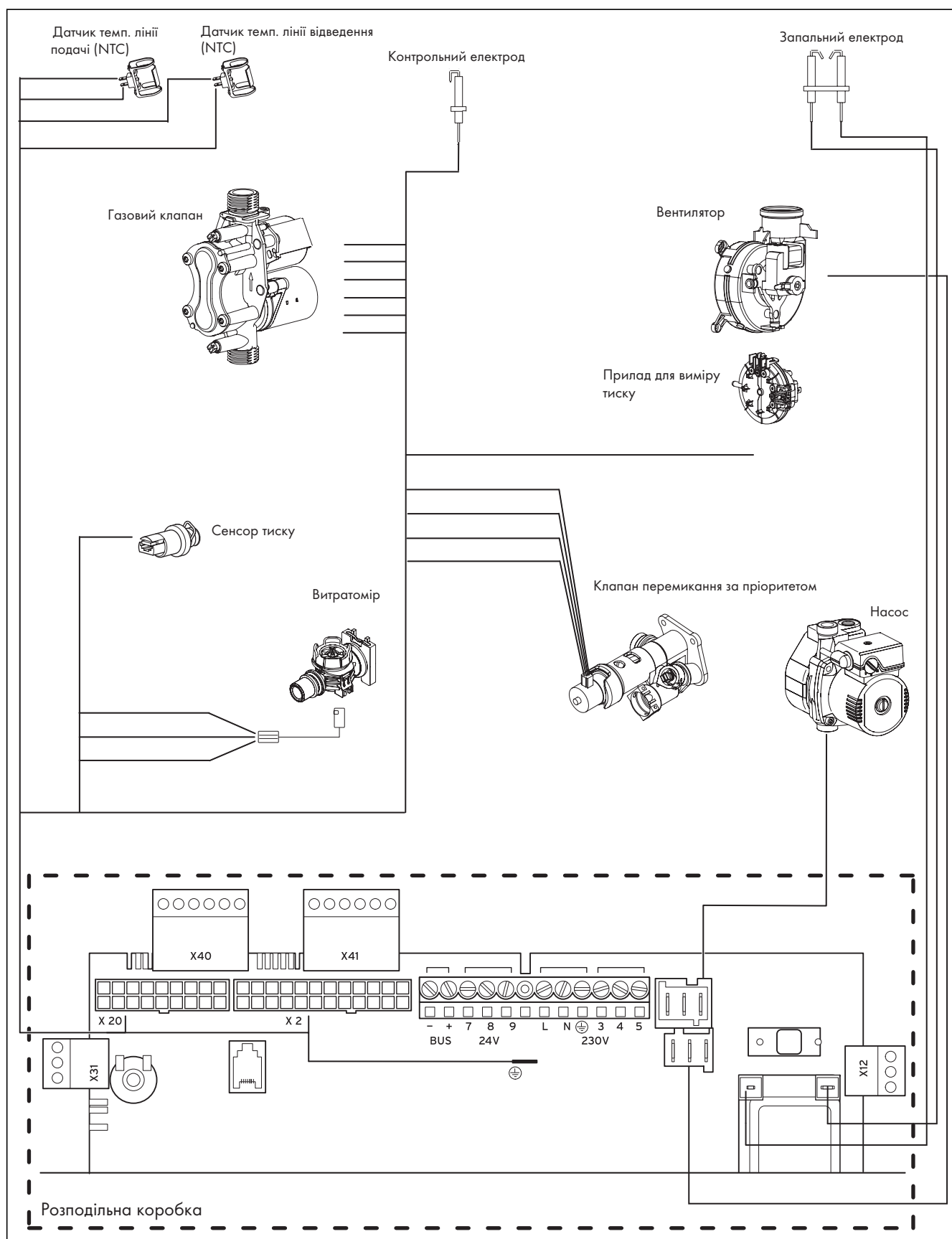
Мал. 5.9 Схема електропроводки turboTEC pro
