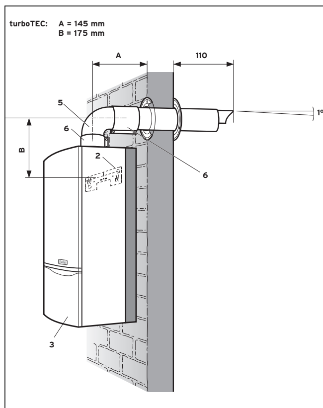
Мал. 4.25 Монтаж приладу (пряма установка)
