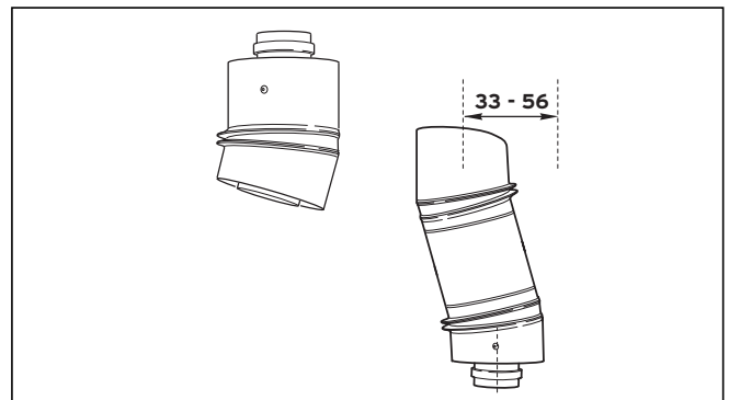
Мал. 4.5 Телескопічний відвід
