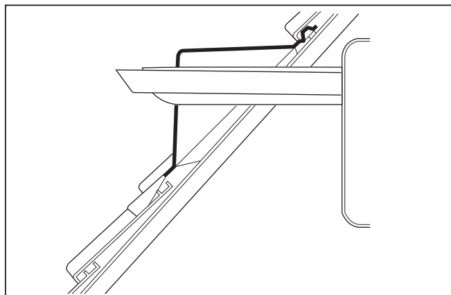
Мал. 5.22 Приклад монтажу горизонтального покрівельного уведення (слухове вікно)
