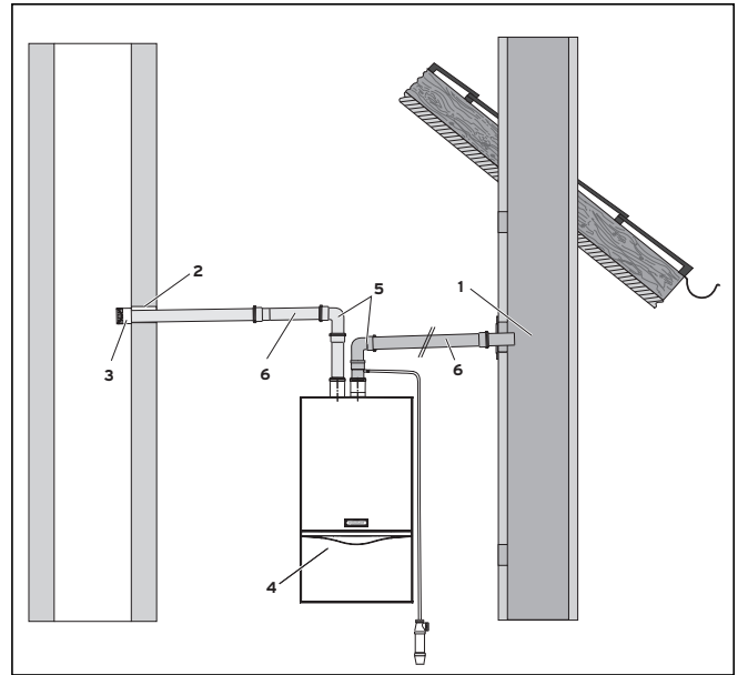
Мал. 6.16 Подача дуттєвого повітря з каналу
