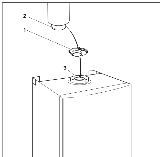
Мал. 5.13 Монтаж заслонок відпрацьованих газів
