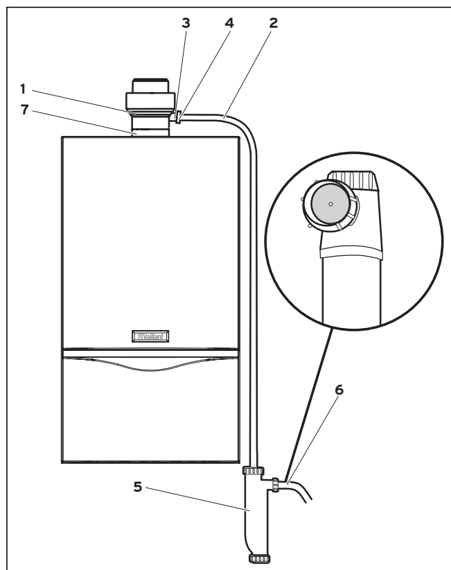
Мал. 5.15 Монтаж перехідника приладу
