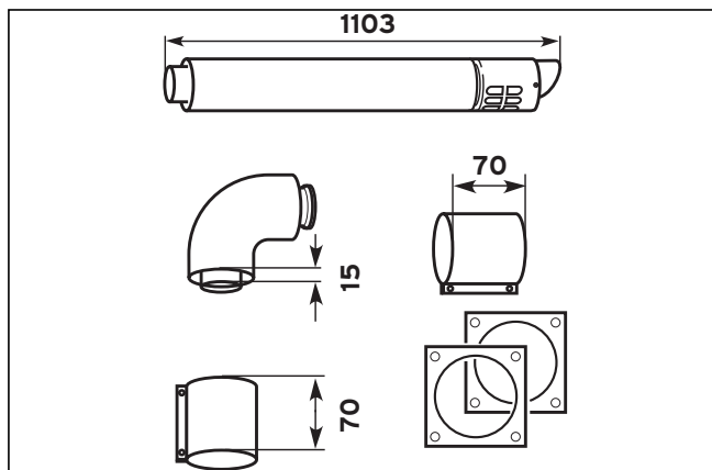
Рис. 5.20 Горизонтальный ввод через стену/кровельный ввод
