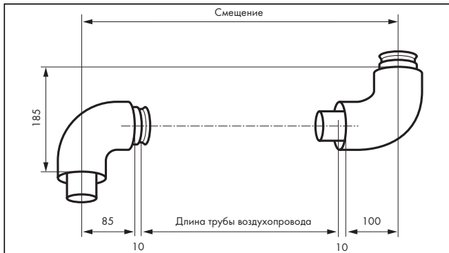
Рис. 4.29 Монтаж колен 90°
