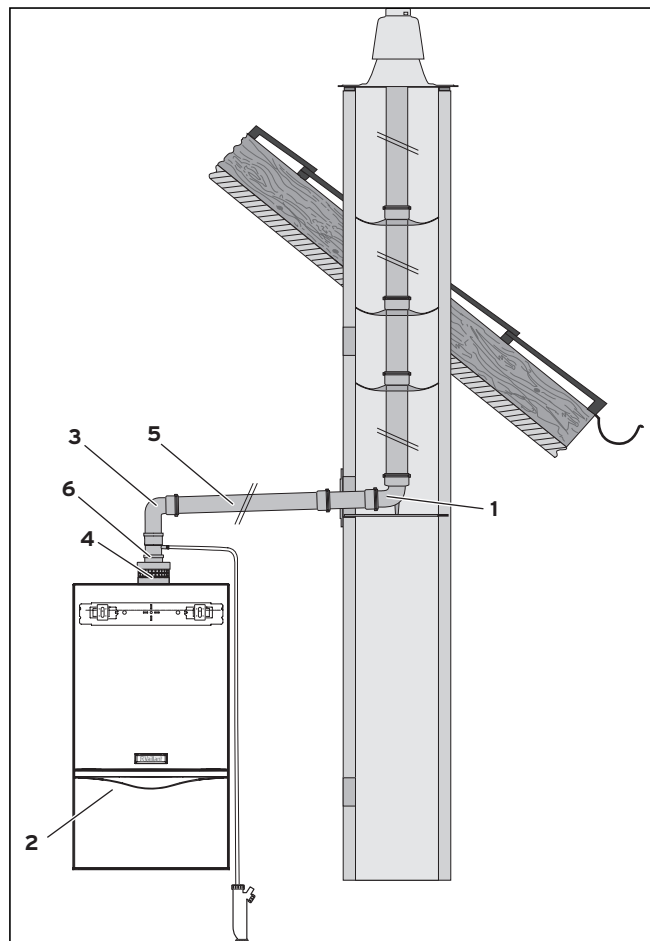
Рис. 6.11 Монтаж
