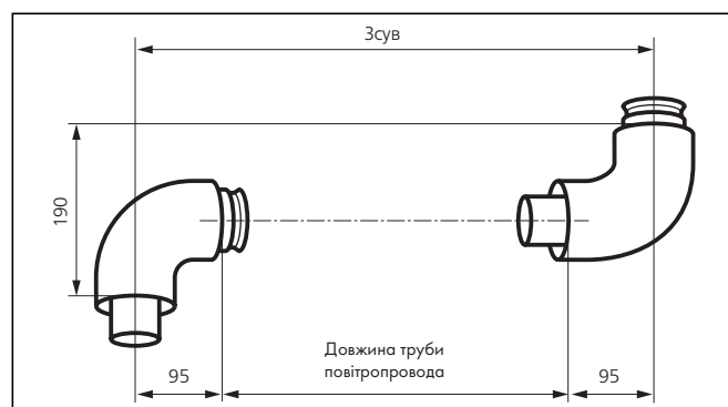
Мал. 5.28 Монтаж колін 87°
