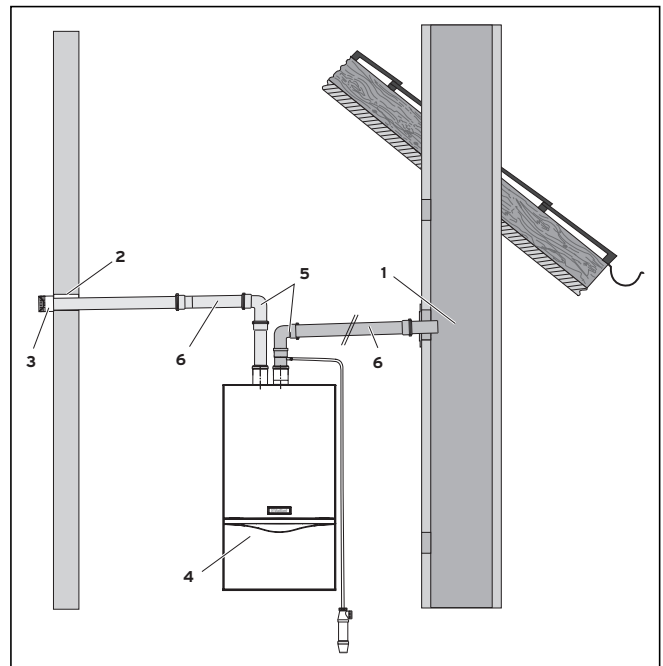
Рис. 6.19 Подача дутьевого воздуха с фасада
