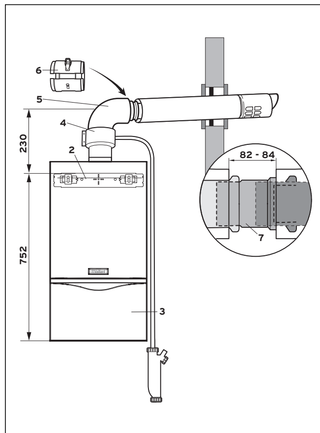
Рис. 5.25 Удаленная установка
