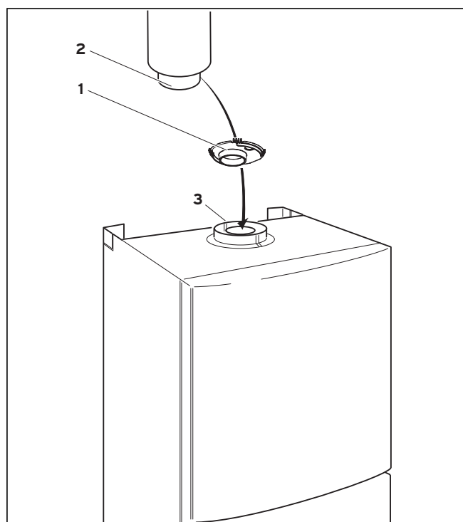
Мал. 6.8 Монтаж труби для відпрацьованих газів
