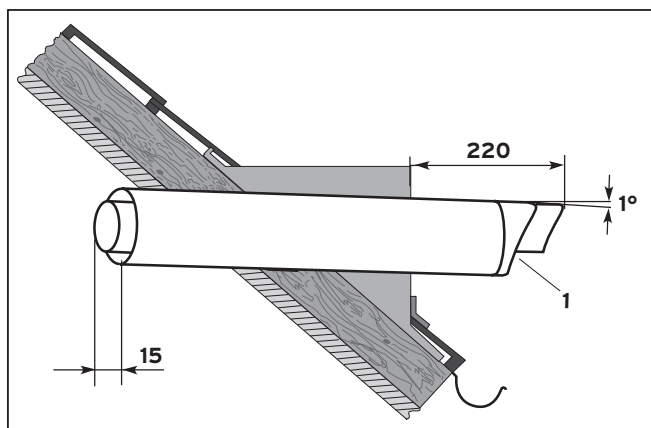
Рис. 5.23 Вмонтирование горизонтального кровельного ввода
