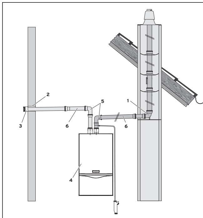
Рис. 6.17 Подача дутьевого воздуха через наружную стену
