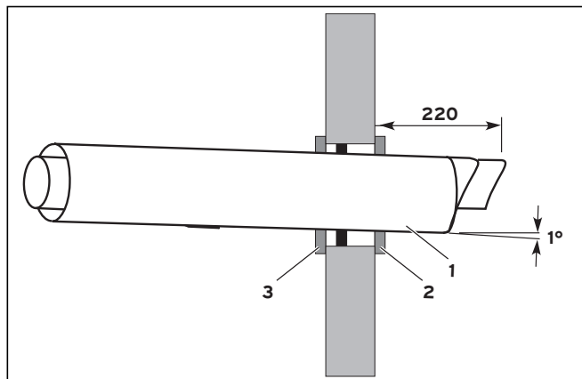
Рис. 5.21 Вмонтирование горизонтального кровельного ввода
