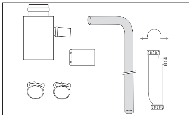
Мал. 4.14 Конденсатовідвідник
