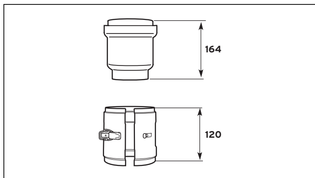
Рис. 5.5 Разделитель, Ø 80/125
