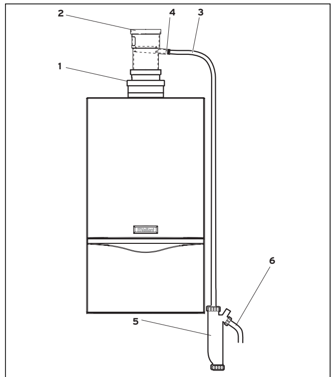
Мал. 6.10 Монтаж сполучного елемента з конденсаторівідвідником
