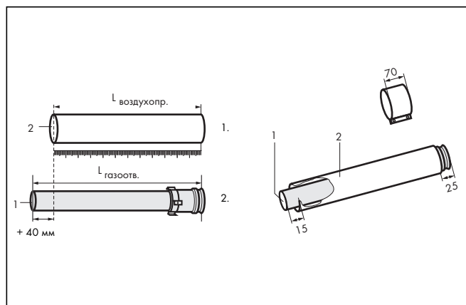
Рис. 5.26 Укорачивание труб
