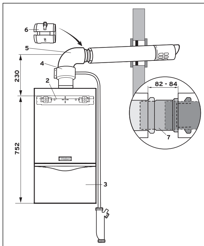
Рис. 5.24 Прямая установка
