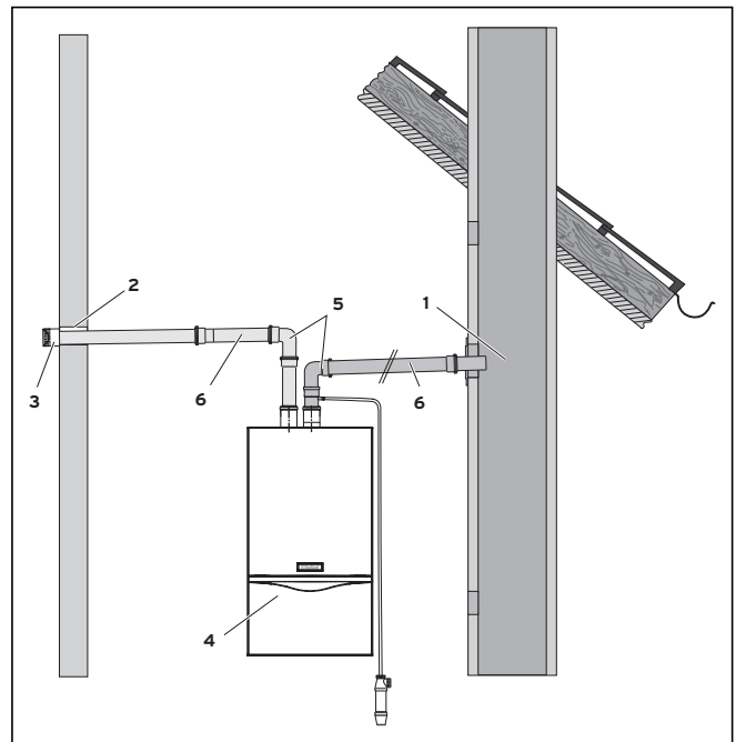
Мал. 6.19 Подача дуттьового повітря з фасаду
