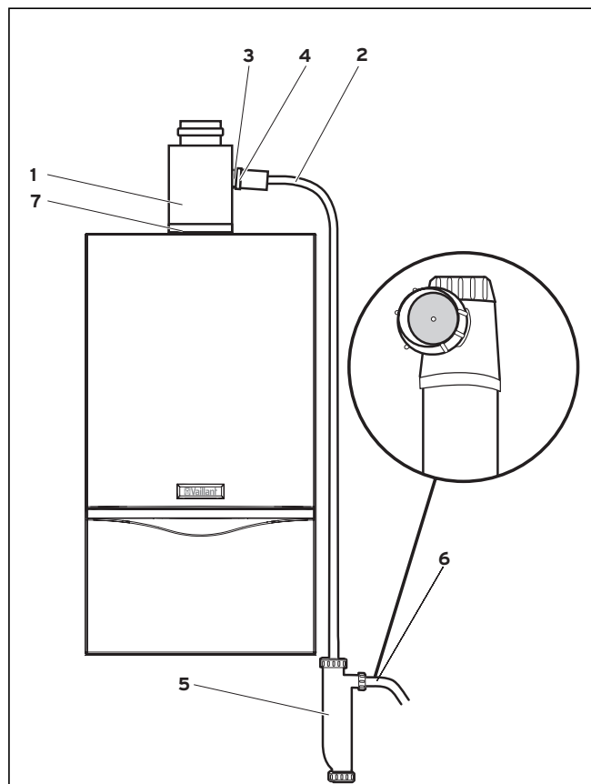
Мал. 4.15 Монтаж перехідника приладу
