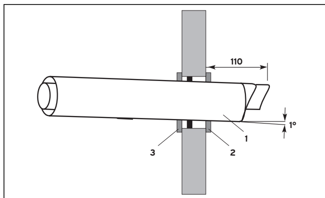
Мал. 4.21 Умонтування горизонтального стінного уведення
